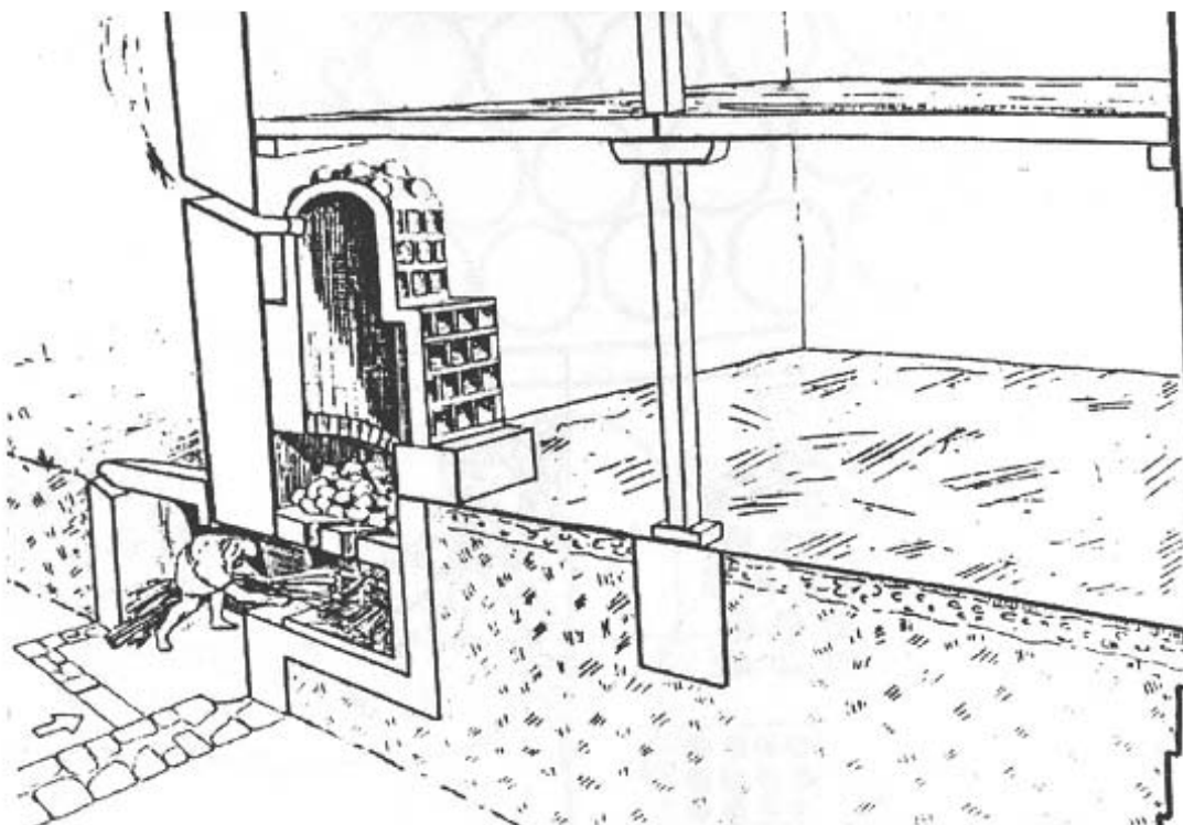
Reconstrucția unui sistem de încălzire, Steinheim Germania (Batariuc)
