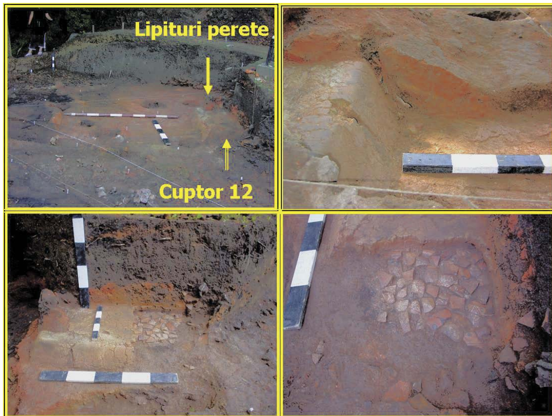
Fetești-La Schit. L 3, cuptorul nr. 12 și detalii constructive
